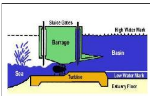
Fig 2: Tidal Barrage
